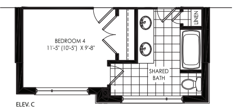
ELEV. C
