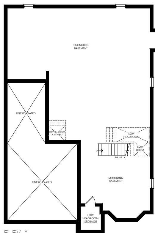
ELEV. A
