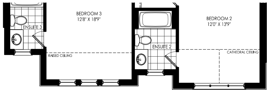
ELEV. B
