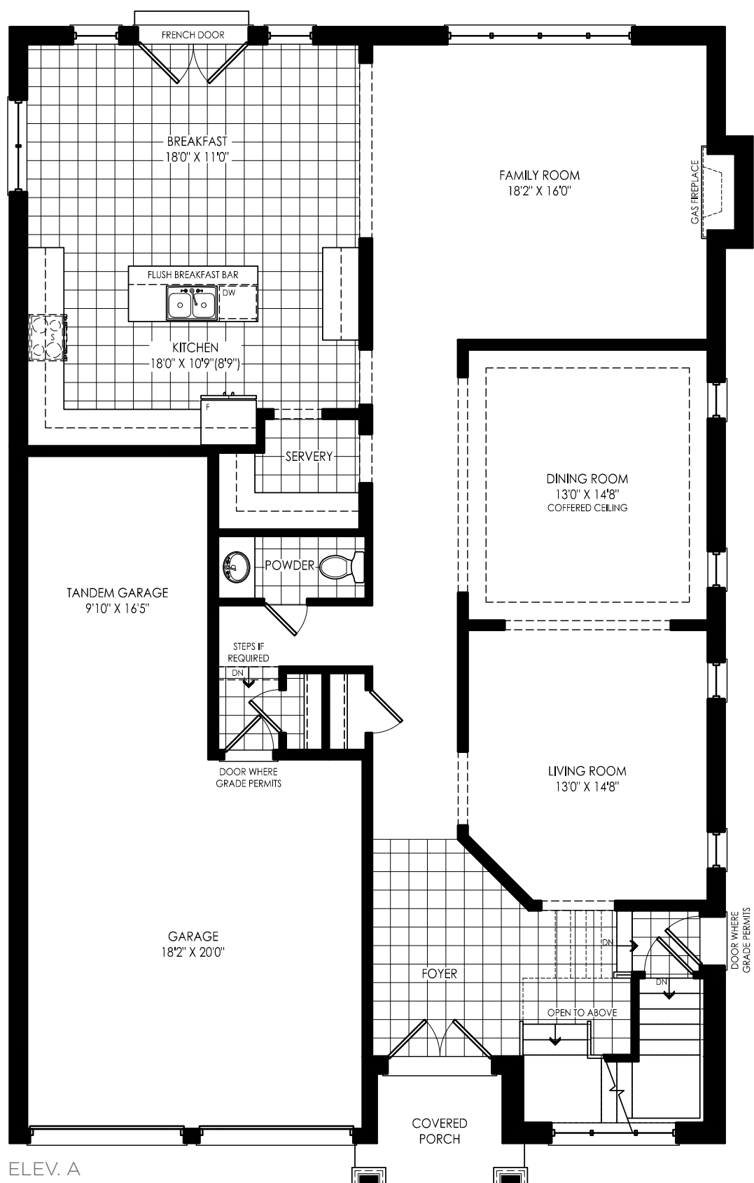
ELEV. A
