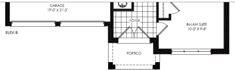
ELEV. B
