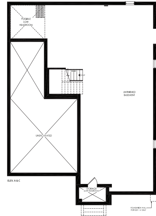
ELEV. A
