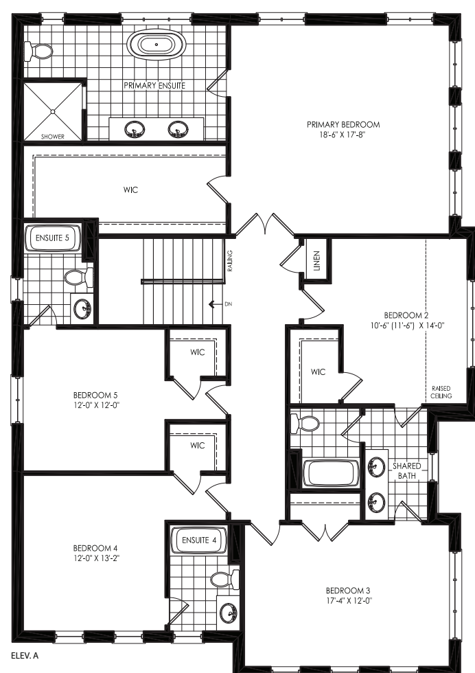
ELEV. A
